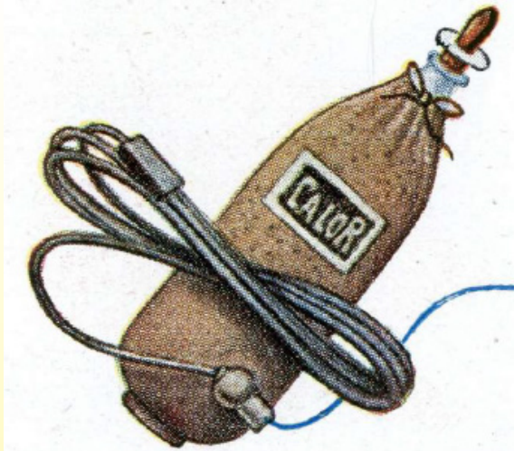
1926 Scaldabiberon flessibile Calor con interruttore sul cavo (Catalog Calor 1926, Ultiheat Museum)
