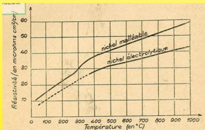
Variazione della resistività del nichel in funzione della temperatura: effetto di autoregolazione. (1945 Modern Electrotechnical Materials, Ultiheat Museum)
