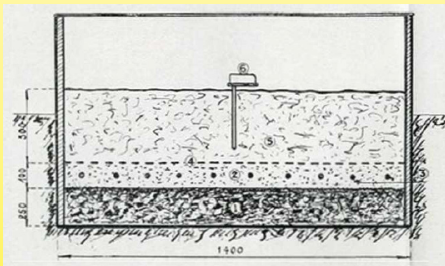
1: scoria, 2: sabbia, 3: cavo riscaldato, 4: rete, 5: terriccio 6: limitatore di temperatura
